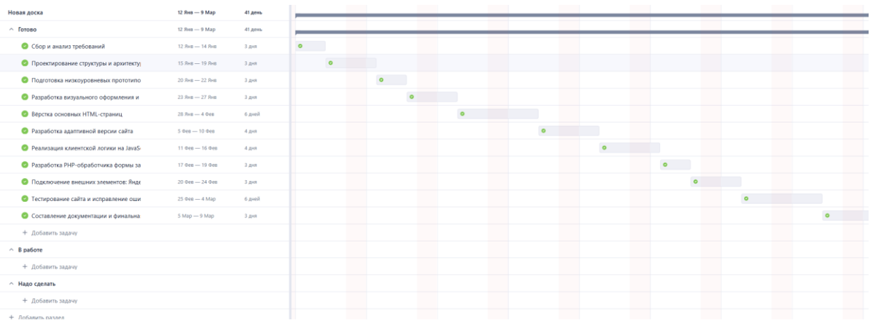
Рисунок 20 – Диаграмма Ганта
