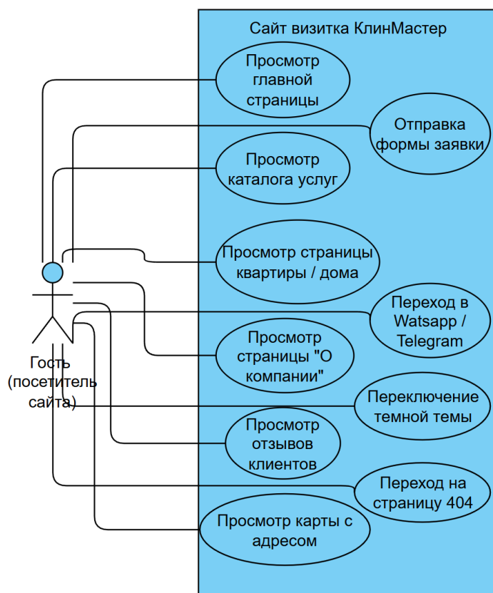
Рисунок 2 – Use Case
